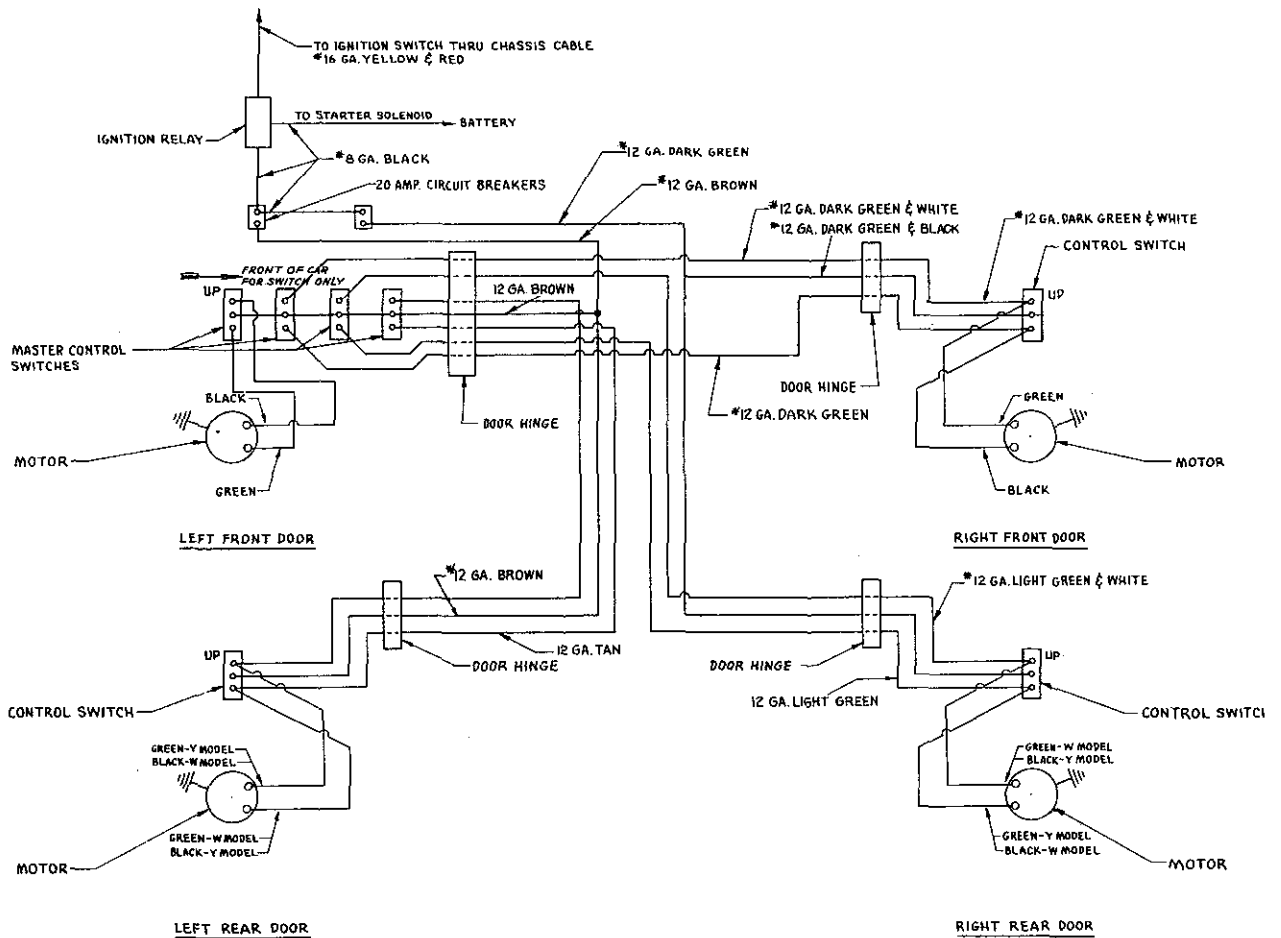
Wiring diagram—4 door sedans FIG. 3 WINDOW LIFT WIRING DIAGRAM
